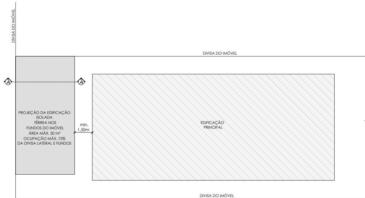
PLANTA BAIXA
